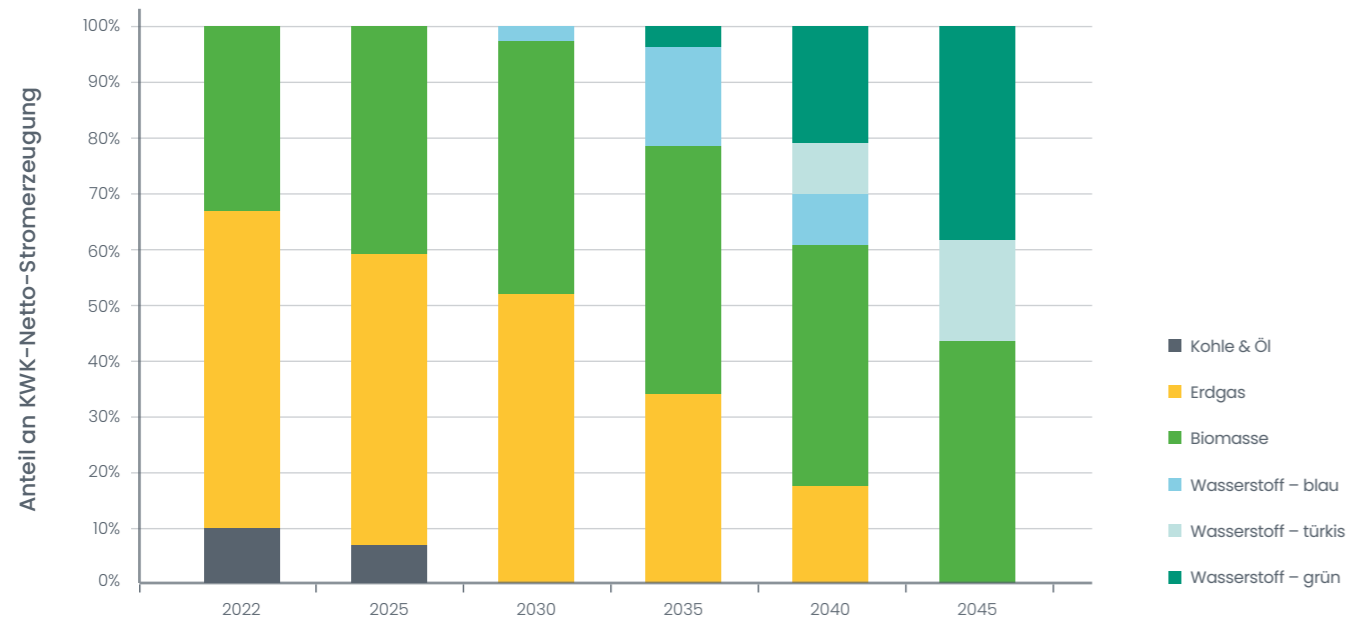
Abbildung 4: Zukünftige Rolle von Wasserstoff als Energieträger in der KWK Quelle: Frontier Economics
